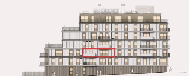
Alçado Sul | South Facade
